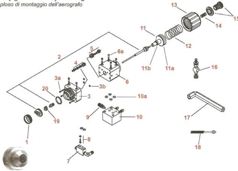
Spray gun assembly drawing Esploso di montaggio dell'aerografo
